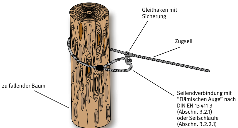
Abb. 15 Direktes Anschlagen mit dem Windenseil am Beispiel eines zu fällenden Baumes
