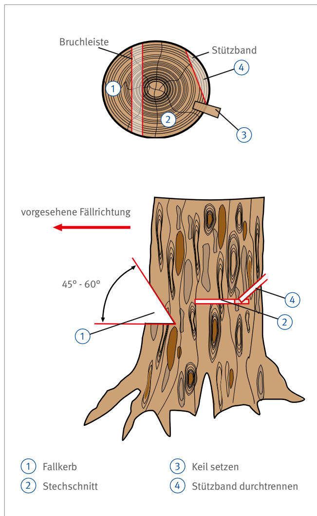
Abb. 78 Fälln mit Stützbandtechnik
