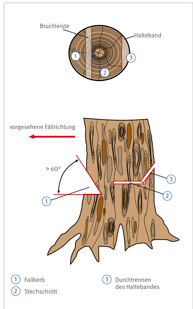
Abb. 79 Fälln mit Haltebandtechnik beim Vorhänger
