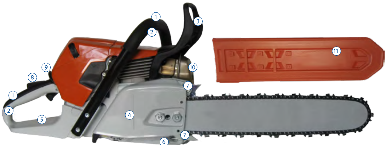
Abb. 23 Motorsäge mit Sicherheitseinrichtungen
