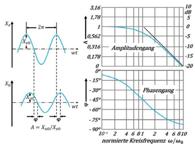
Abb. 3.8.5 Frequenzgang
