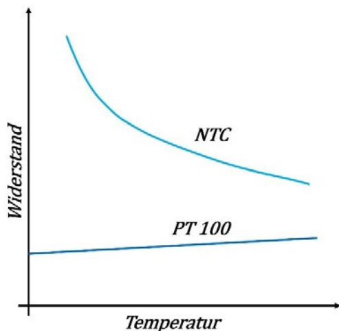
Abb. 3.8.3 Statische Kennlinien von Temperaturfühlern
