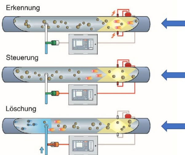
Abb. 3.9.2 Bestandteile und Wirkungsweise einer Funkendetektions- und -löschanlage
