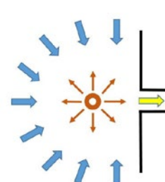
Offene Erfassungseinrichtung in Saugrohr-Ausführung
