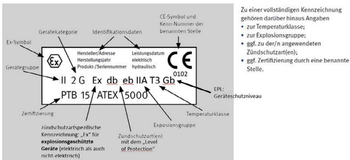
Abb. 5.3.3 Beispiel einer Kennzeichnung nach ATEX-Richtlinie (Richtlinie 2014/34/EU, Anhang II)
