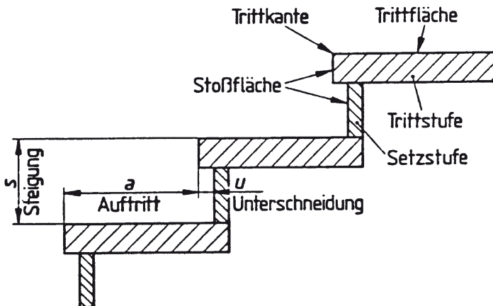
Bezeichnung von Treppenteilen
