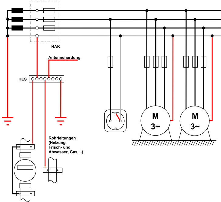
Abb. 55 TN-C-System
