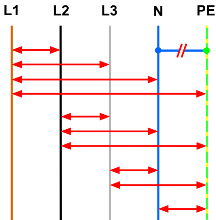
Abb. 21 Isolationswiderstandsmessung, z. B. in feuer- oder explosions- gefährdeten Bereichen
