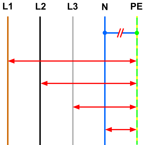
Abb. 19 Isolationswiderstandsmessung; Einzelmessung
