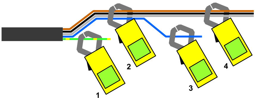
Abb. 23 Bestimmung der Ströme in Schutzleiter und Neutraleiter (1 I_{PE} , 2 I_{Diff} , 3 I_{Nist} , 4 I_{Bedarf} (demand))
