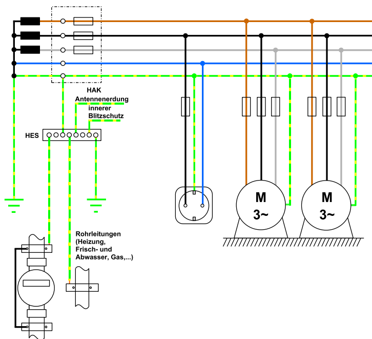
Abb. 56 TN-S-System
