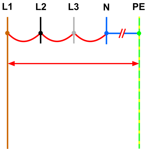
Abb. 20 Isolationswiderstandsmessung; Mit gebrückten aktiven Leitern
