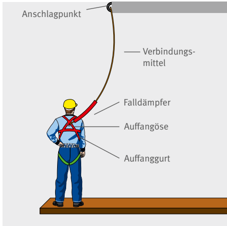
Abb. 17 Auffangsystem mit Falldämpfer: Der Auffanggurt wird über ein Verbindungs-mittel und einen Falldämpfer mit einem Anschlagpunkt am Mast verbunden. Der Anschlagpunkt liegt möglichst oberhalb des Arbeitsplatzes.
