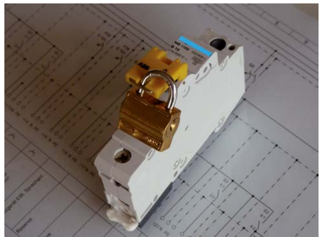
Bild 5-12: Leitungsschutzschalter mit Abschießvorrichtung sichert gegen Wiedereinschalten
