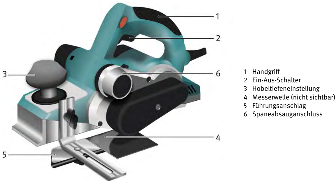
Abb. 3.3.3-01 Elektrohobelmachine
