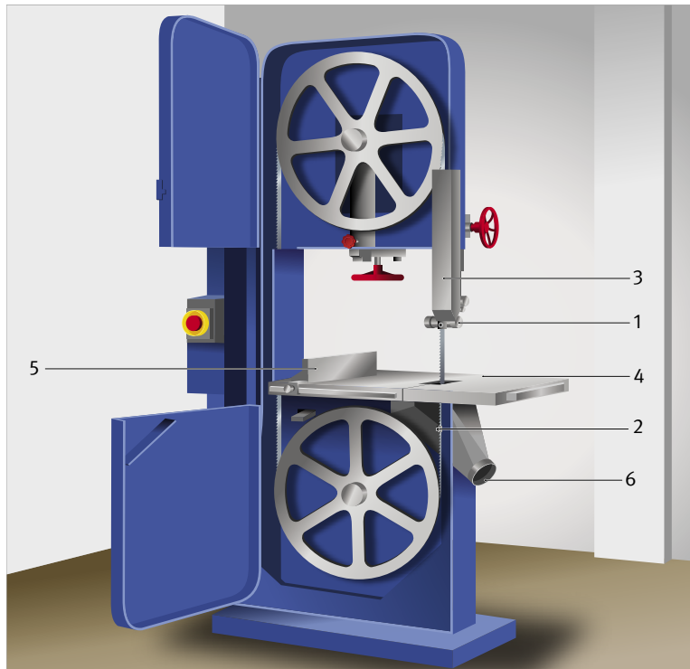
Abb. 3.1.6-01 Tischbandsägemaschine
