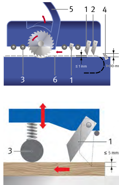
Abb. 3.1.14-02 Anordnung der Rückschlag- und Splitterfangeinrichtung
