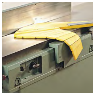
Abb. 3.1.9-04 Gliederchwingschutz für Altmaschinen
