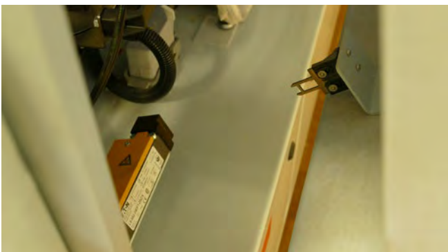
Abb. 3.1.12-03 Elektrisch verriegelte bewegliche Schutzeinrichtung mit Zuhaltfunktion für Kapp- und Bündigfräsaggregate
