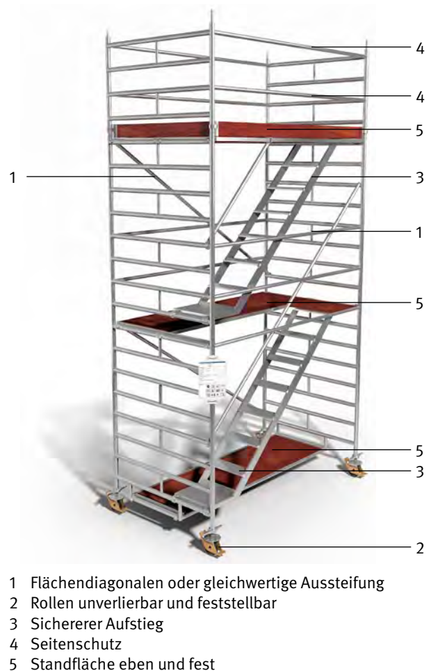
Abb. 3.5.3-03 Fahrbare Arbeitsbühne
