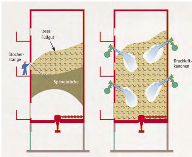
Abb. 3.4.2-03 Druckluftkanonen
