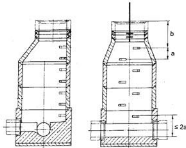
Bild 1: Schacht mit senkrechtem Steiggang
